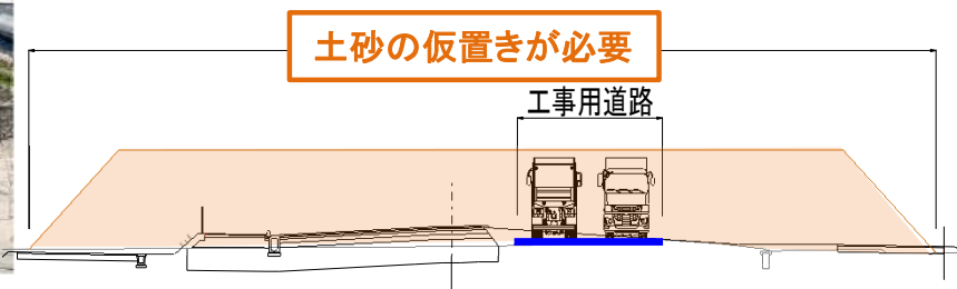
ステップ1 (工事用道路や本線盛土を造るため、土砂の仮置きが必要)
