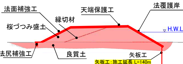
標準横断面図(堤防復旧箇所)
