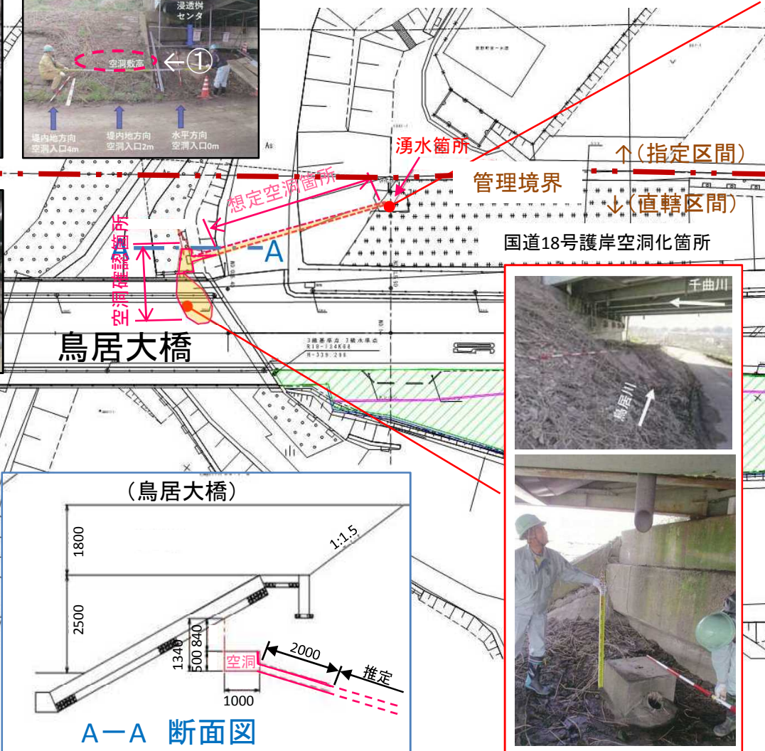
鳥居大橋下路面排水浸透樹
