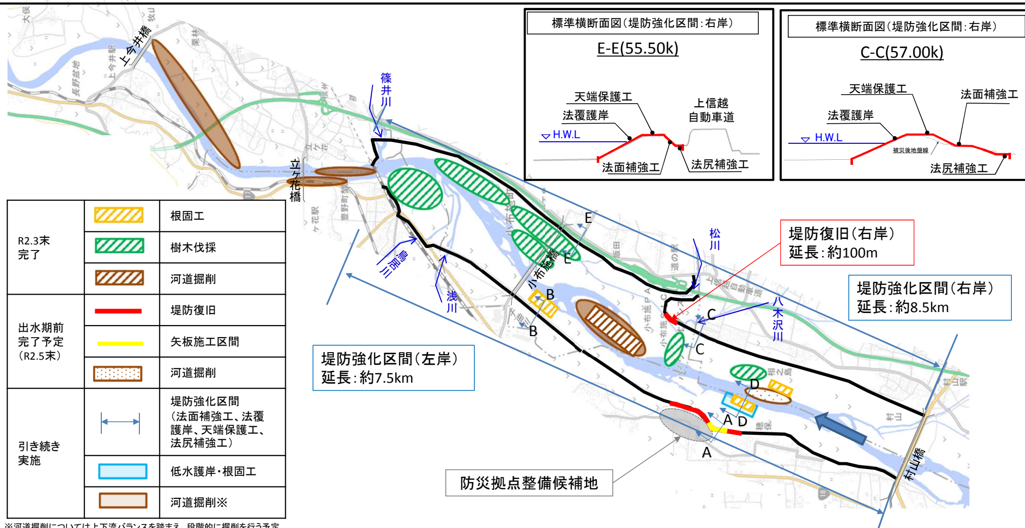
標準横断面図(堤防強化区間:左岸)
